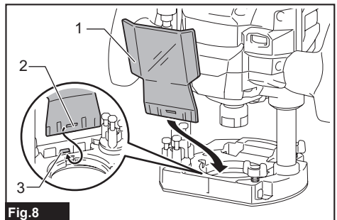
Fig. 8 ► 1. Chip deflector 2. Hole 3. Protrusion
